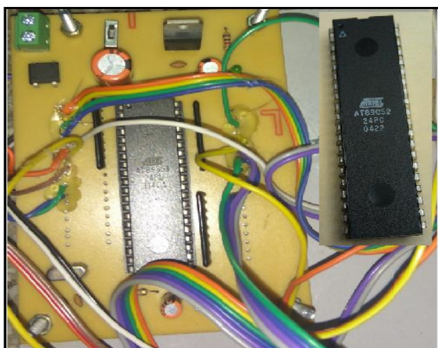
Fig6 AT89C51 Controller & It’s Circuitry
